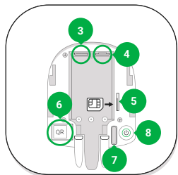
3 - Роз'єм підключення кабелю живлення. 4 - Роз'єм підключення кабелю Ethernet. 5 - Слот карти стільникового оператора (формату Micro-SIM). 6 - QR код. 7 - Кнопка тампера. 8 - Кнопка увімкнення / вимкнення.
