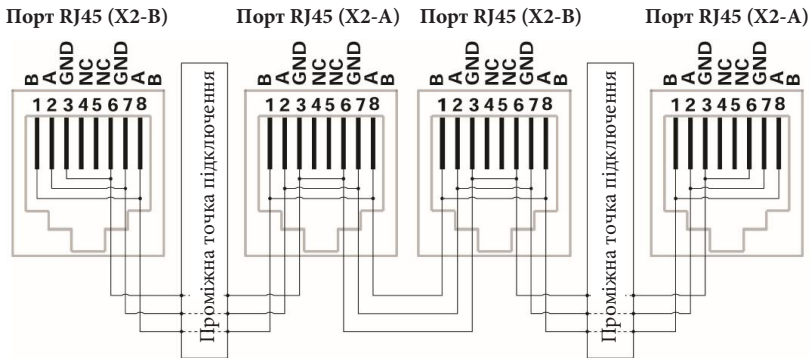
Схема підключення паралельних кабелів RS485
