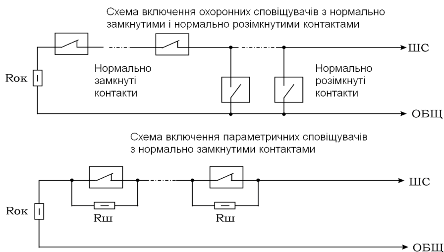
Рисунок 3 – Схеми включення сповіщувачів
