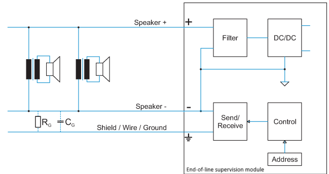
Принципиальная схема
